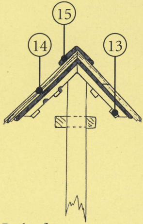
Dachaufbau
